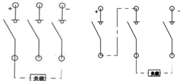
3P 外形接线图(DC500V)
